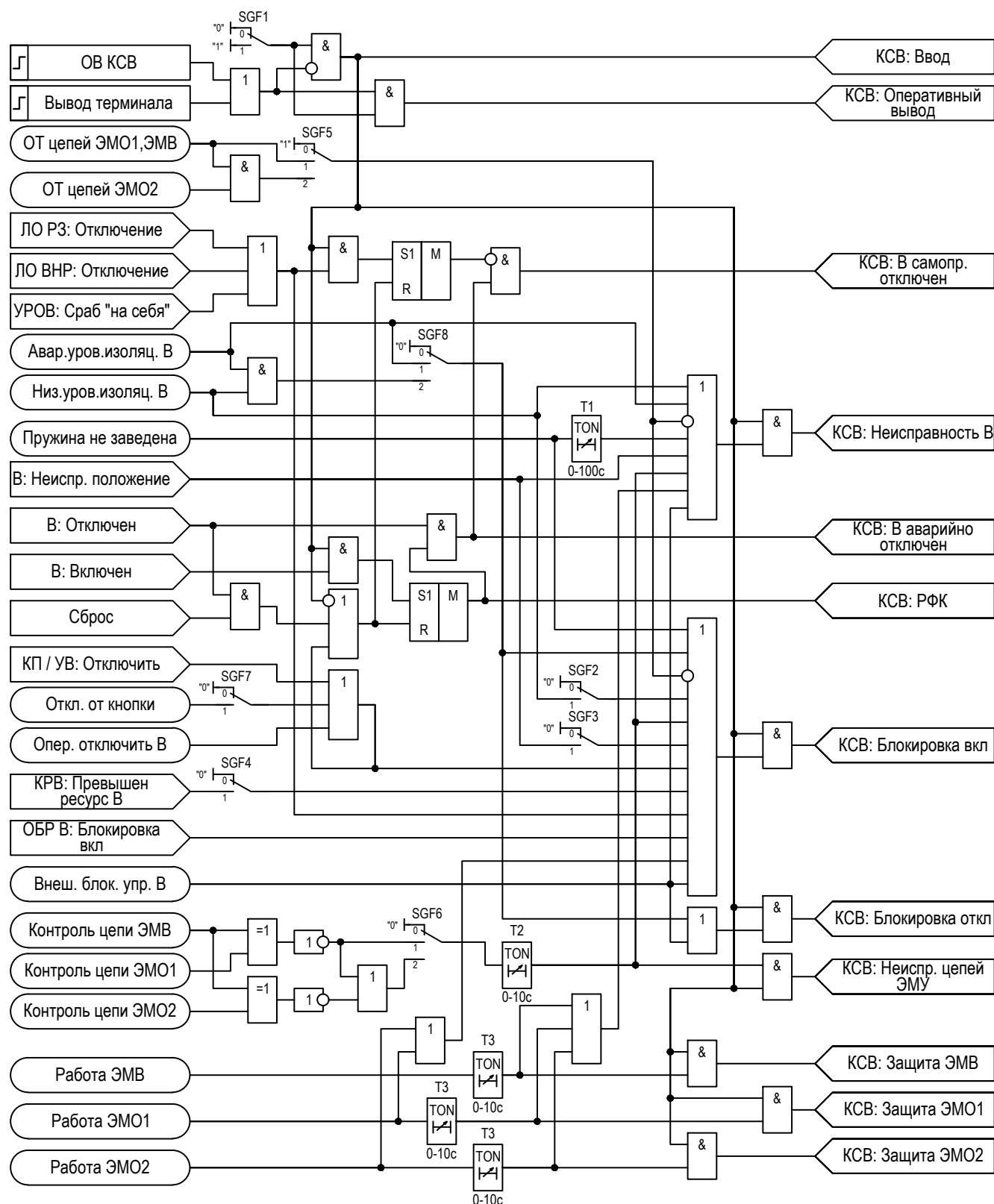
Рисунок 2.68 – Функциональная схема «КСВ»
